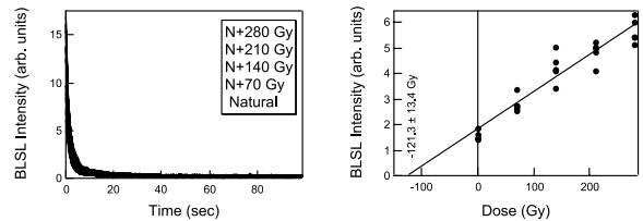
図7-1 BLSL測定による石英微粒子の等価線量評価。左：BLSL減衰曲線、右：生長曲線。BLSL測定では、8~14秒間のルミネッセンス強度を積算して生長曲線を作成した。生長曲線は、最小二乗法で直線回帰を行い、直線を外挿して等価線量 ( 121.3 \pm 13.4 Gy) を求めた。
